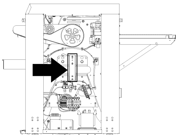
Transportno osiguranje na desnom bočnom nosaču.
