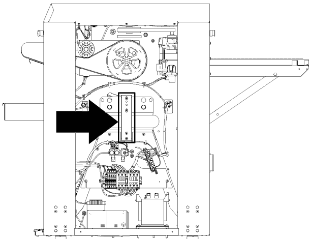
Transportsicherung im rechten Seitenständer.
